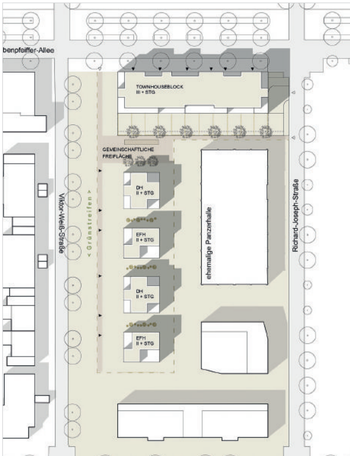
Lageplan
